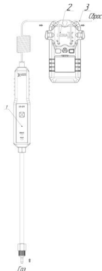
Рисунок Д.2 – Схема соединения моторизированного насоса и газоанализатора 1- Насос; 2 – Калибровочная насадка; 3– Сброс.
