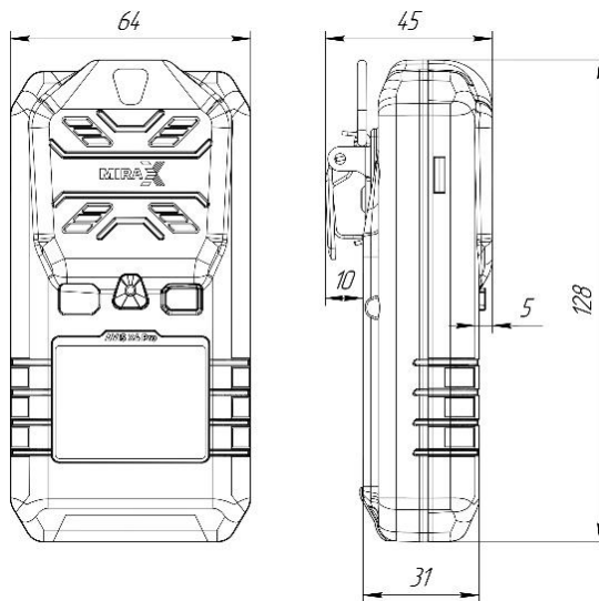
Рисунок 1 – Габаритные размеры газоанализатора
